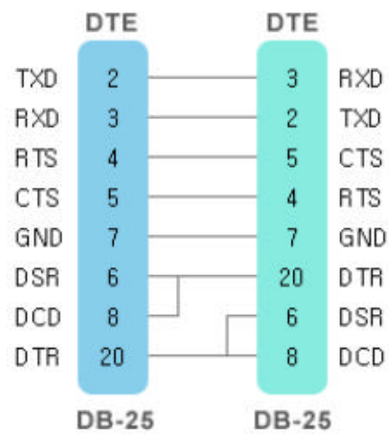
DTE to DTE 7 Wire Cables
