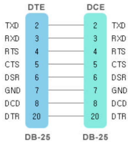
DTE to DCE 8 Wire Cables
